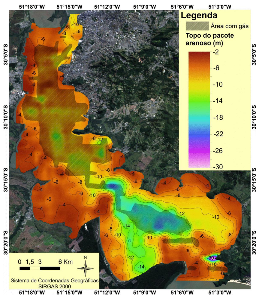
Figura 37: mapa do Topo do Pacote Sedimentar Fonte: Relatório BELOV N°01.HID.021/18-RE.001- R0.
